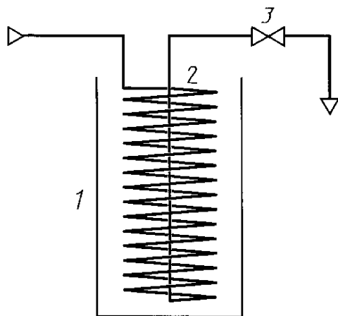
1 — сосуд для охлаждающей смеси; 2 — змеевик; 3 — игльчатый клапан
